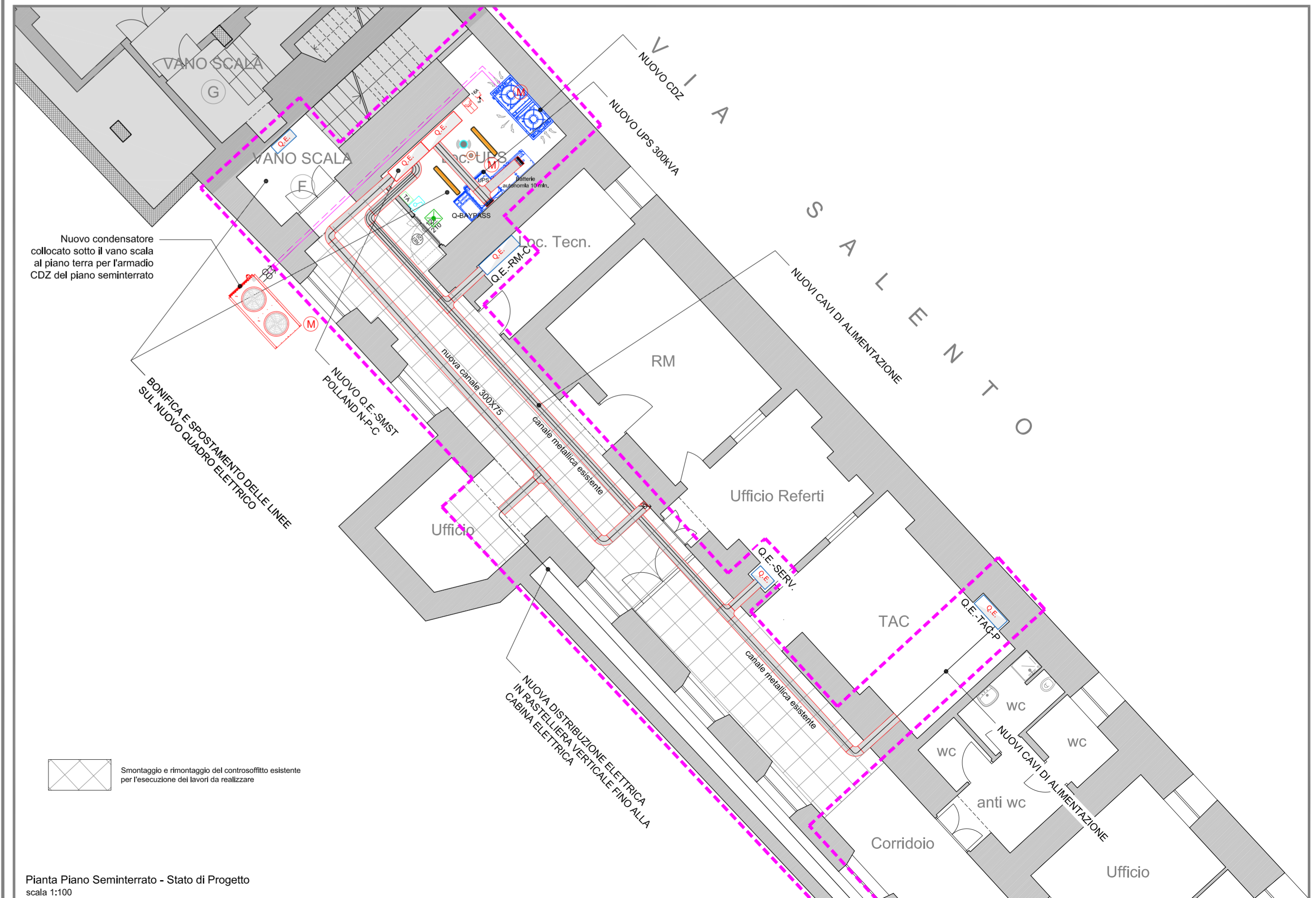
Pianta Piano Seminterrato - Stato di Attuale scala 1:100
